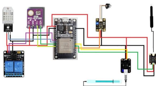
Gambar 1. Rangkain IoT
