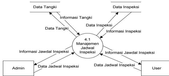
Gambar 3.8 DFD Level 2 Proses Manajemen Jadwal Inspeksi
