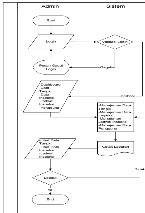
Gambar 3.1 Flowchart Sistem Informasi Inspeksi Tangki
