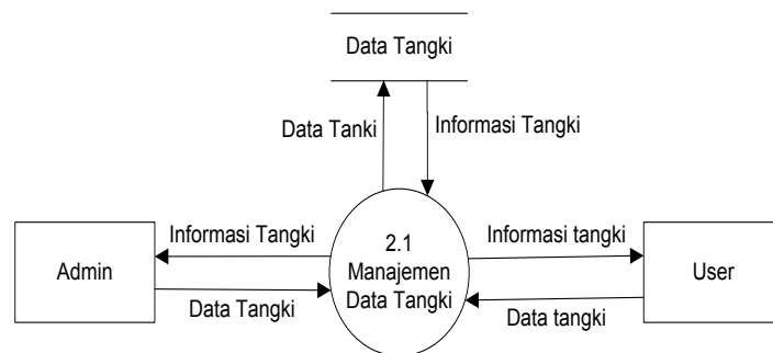
Gambar 3.6 DFD Level 2 Proses Manajemen Data Tangki
