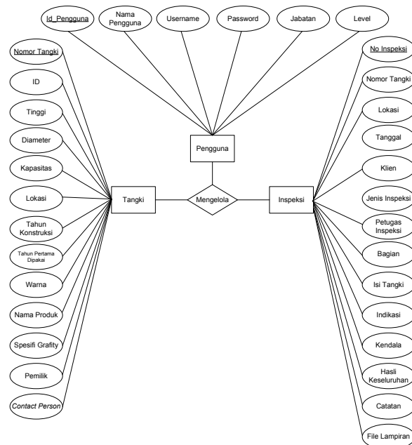
Gambar 3.10 ERD Sistem Informasi Inspeksi Tangki
