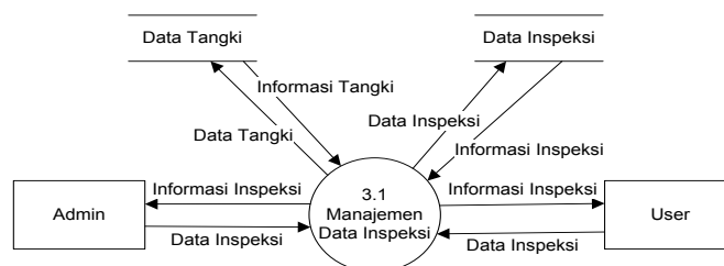
Gambar 3.7 DFD Level 2 Proses Manajemen Data Inspeksi
