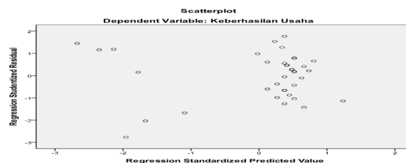
Gambar 1. Hasil Uji Heteroskedastisitas
