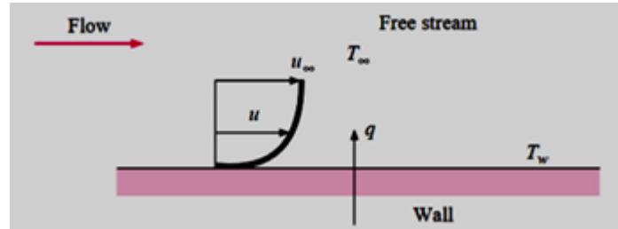
Gambar. 6 Perpindahan Kalor Konveksi Dari Suatu Plat
