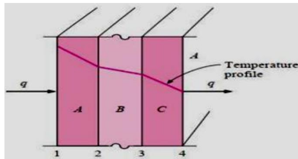
Gambar 5. Perpindahan kalor melalui dinding
