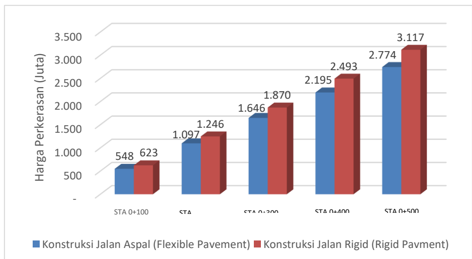
Gambar 4. Grafik Pernadingan Biaya Konstruksi Jalan Aspal ( Flexible Pavement ) Dengan Biaya Konstruksi Jalan Rigid ( Rigid Pavement )
